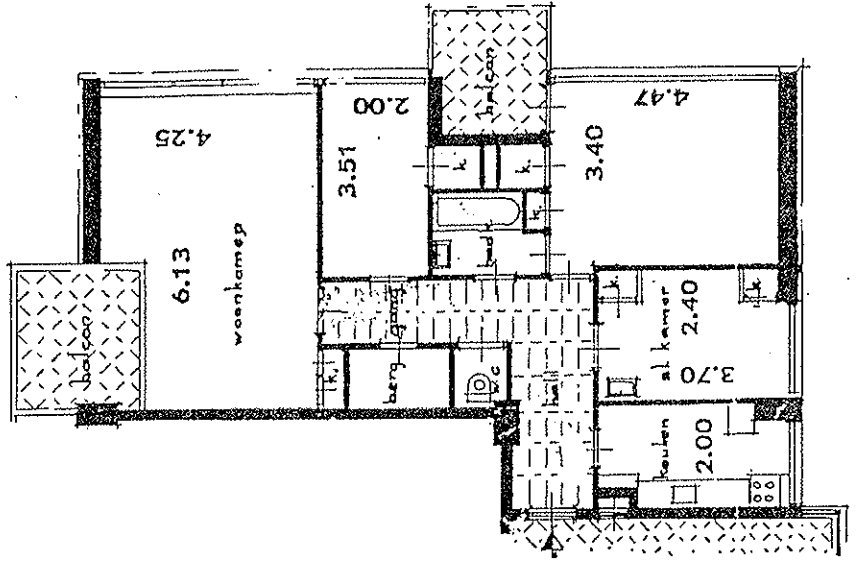
Kopwoning - 4 kamers
