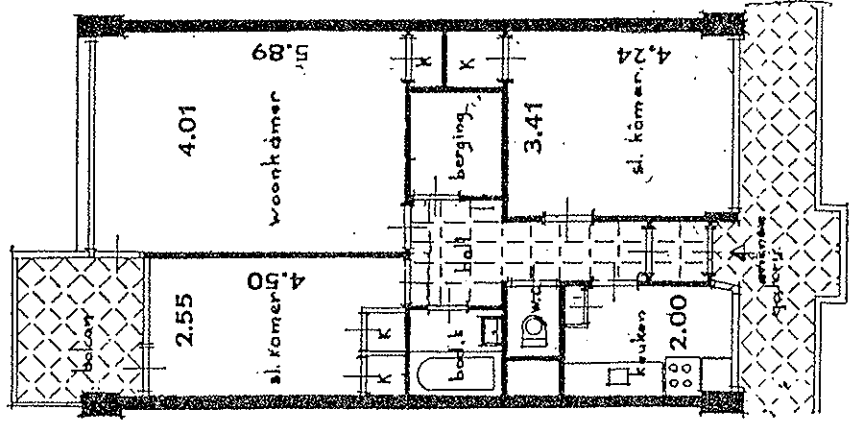
Normal-woning - 3 kamers
